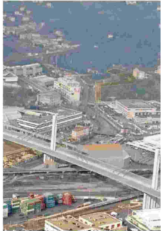
Il progetto del ponte della Gronda a Bolzaneto
